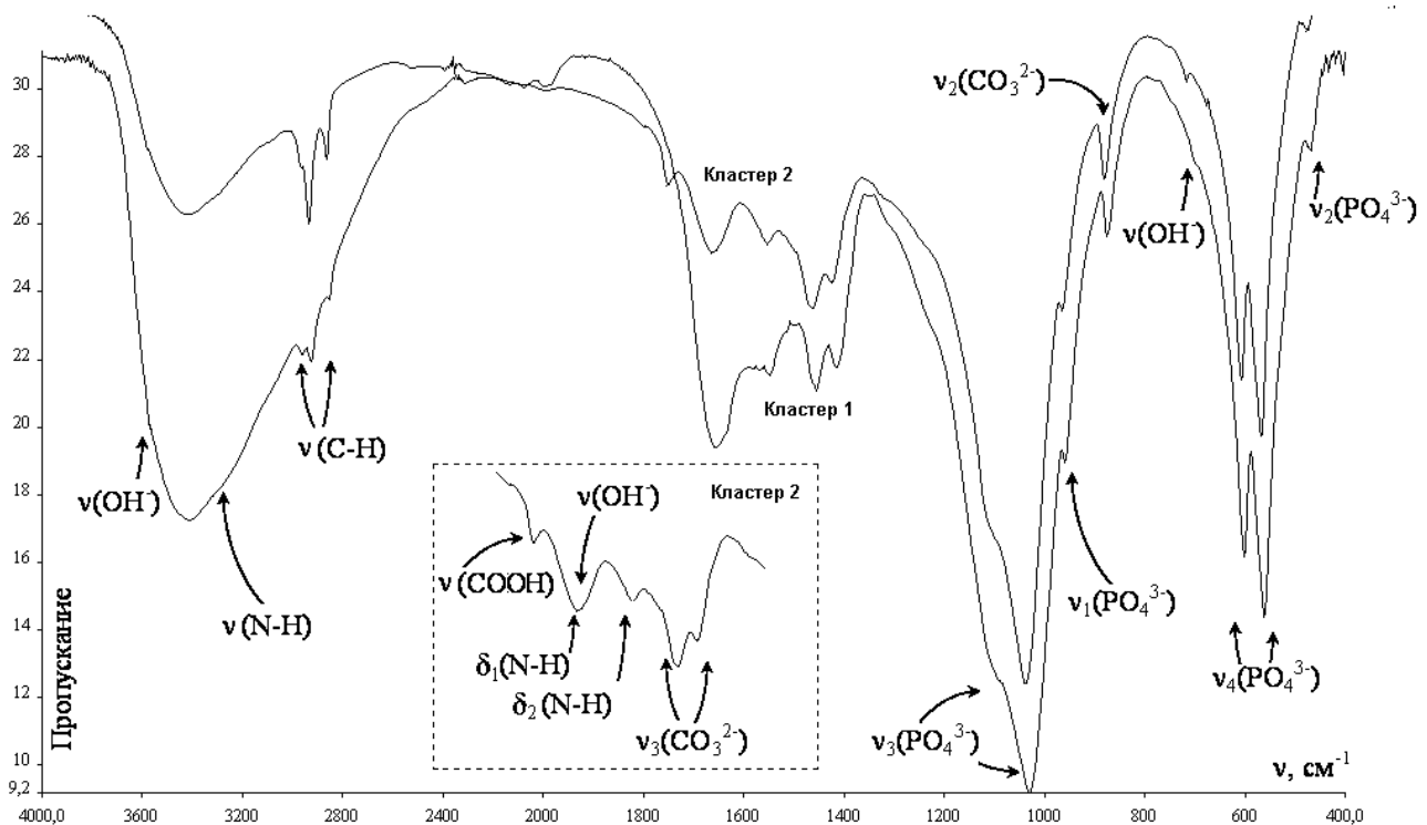
Рисунок 3. ИК-спектры образцов СК.
